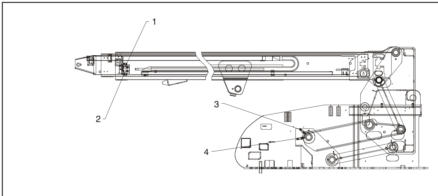
图 2-5. 水平和载重能力限制开关- 第 1 页，共 2 页
