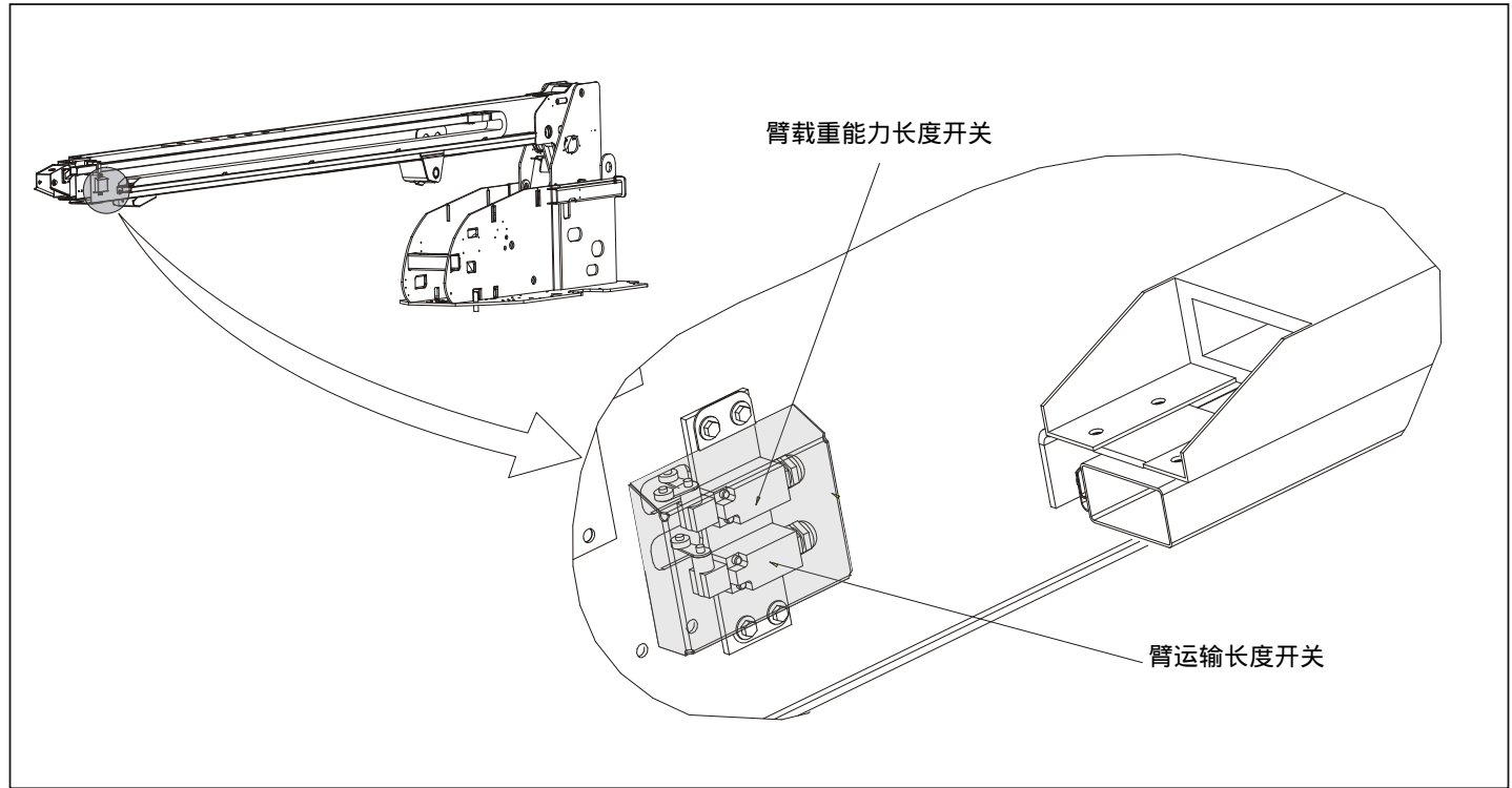
图 2-8. 限位和停止开关 - 第 2 页, 共 2 页
