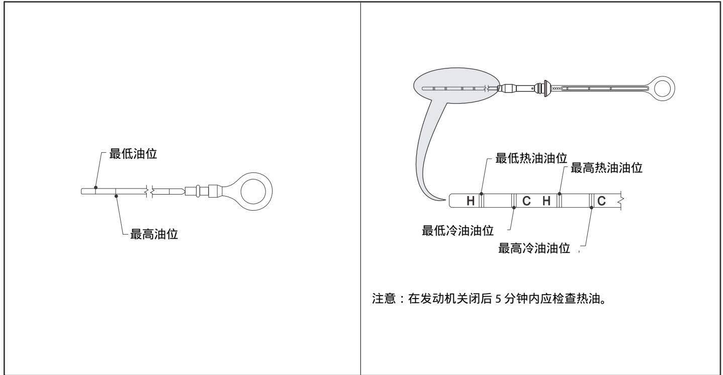
图 6-7. Deutz 2011 发动机量油尺
