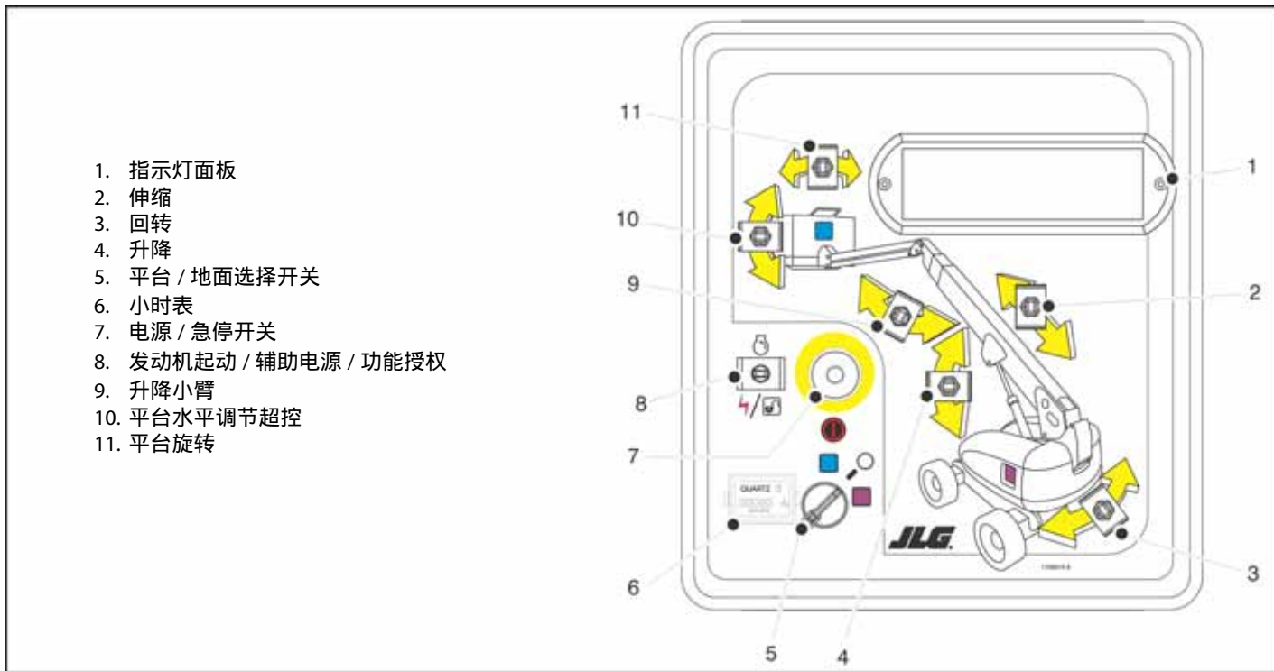
图 3-1. 地面控制台 - 860SJ
