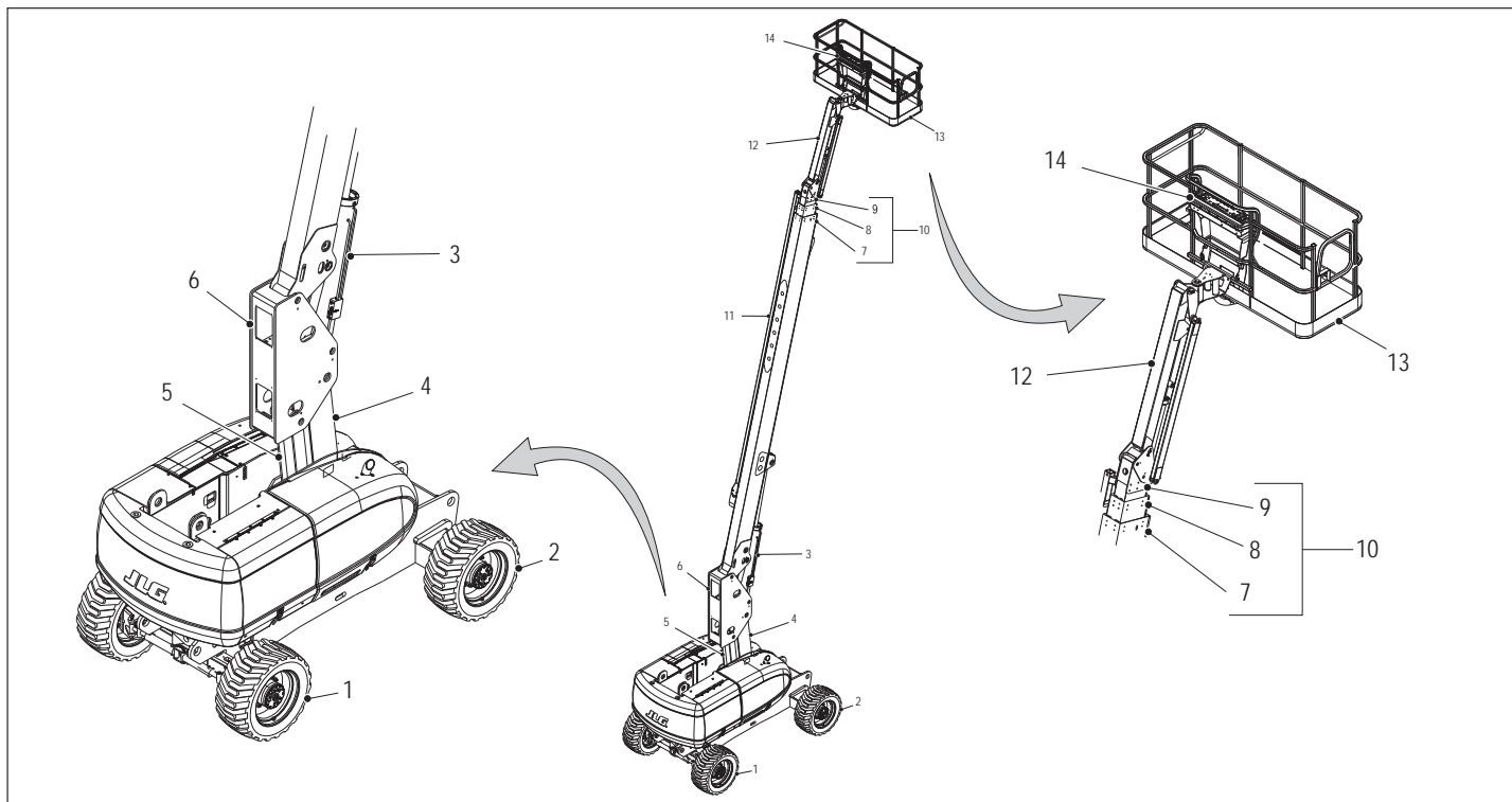
图 2-1. 基本部件名称 - 第 1 页, 共 2 页
