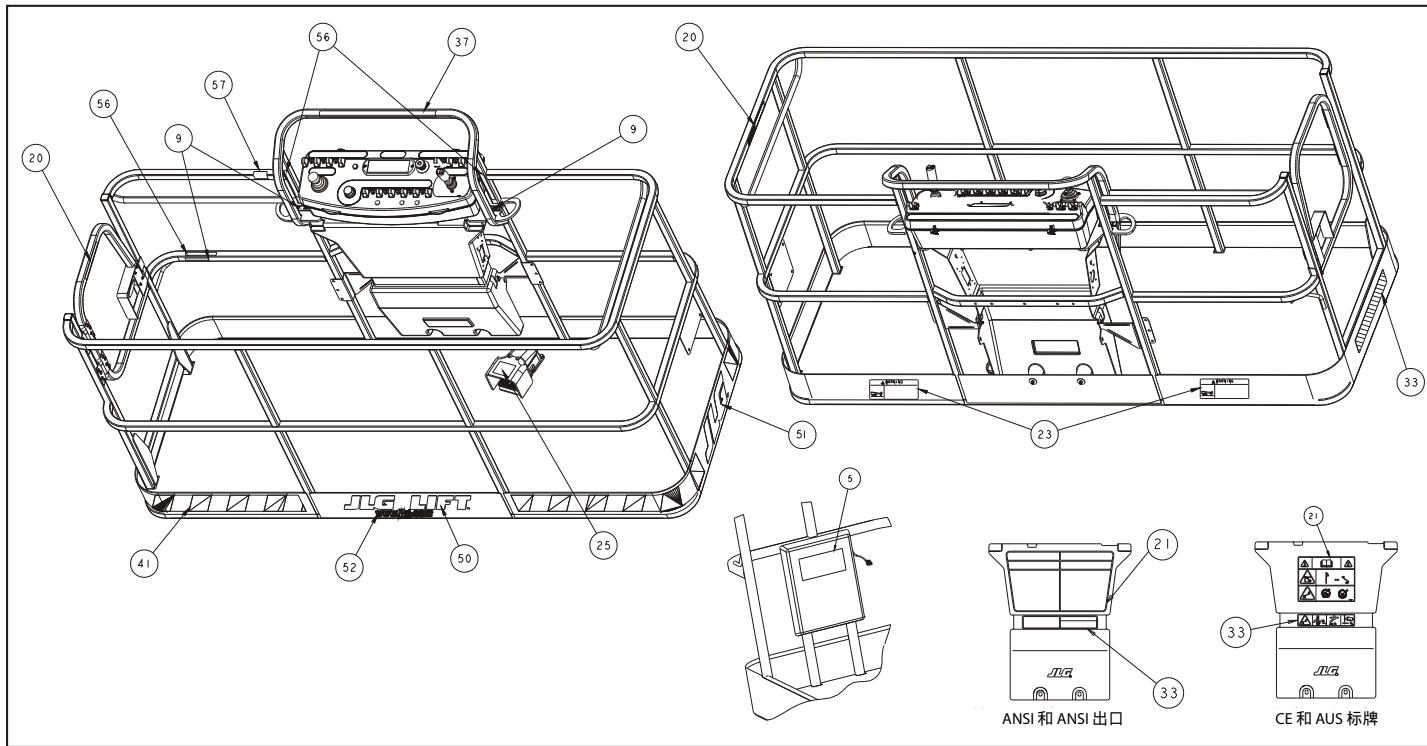
图 4-11. 标志位置 - 第 5 页，共 5 页
