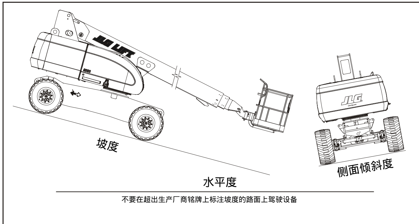
图 4-3. 坡度和侧面倾斜度
