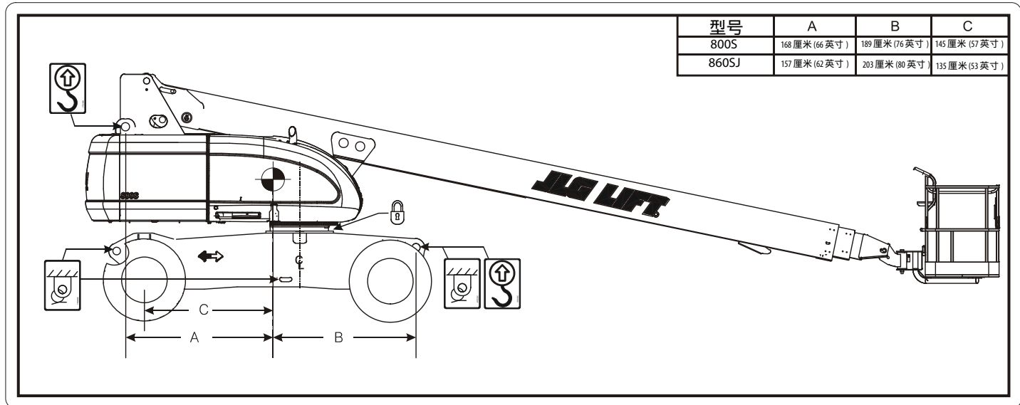
图 4-6. 举升和捆绑图
