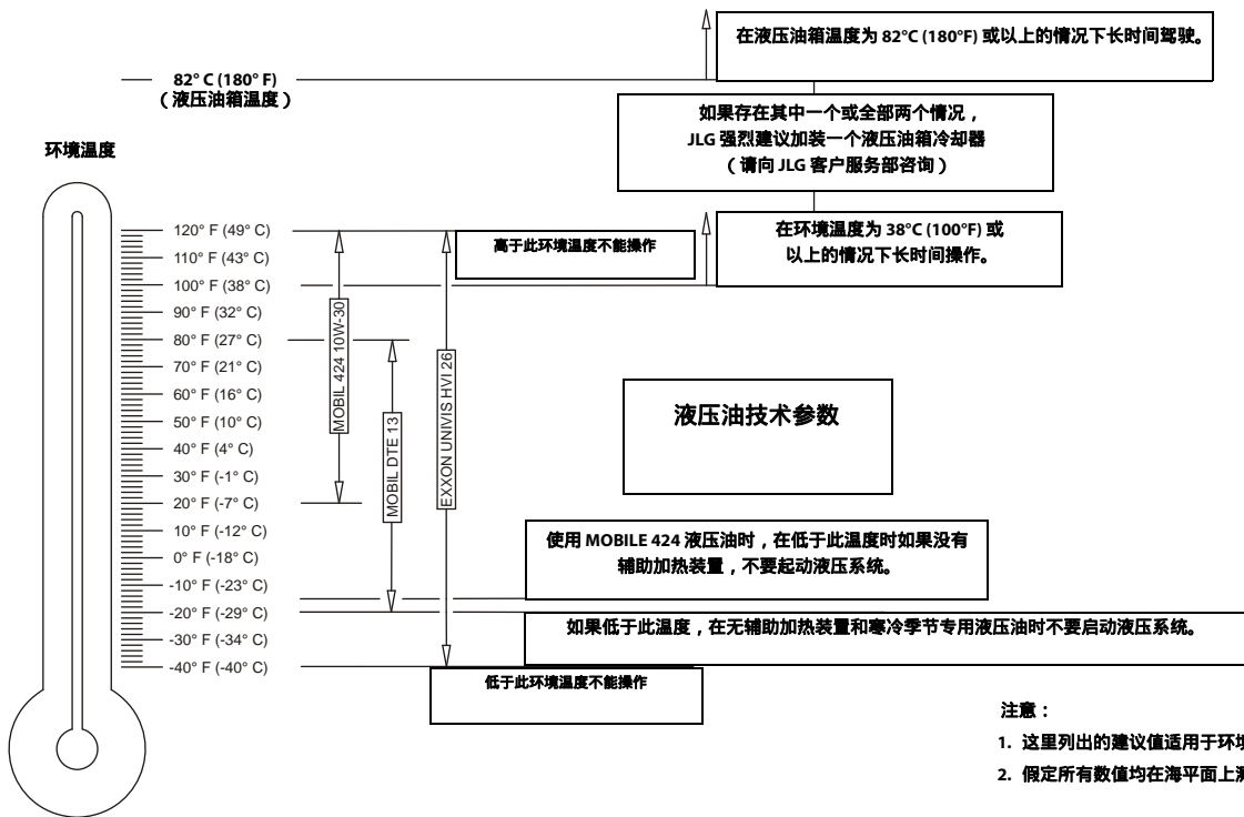
图 6-5. 发动机工作温度技术参数 - GM - 第 2 页, 共 2 页
