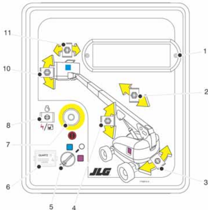
图 3-1. 地面控制台 - 800S
