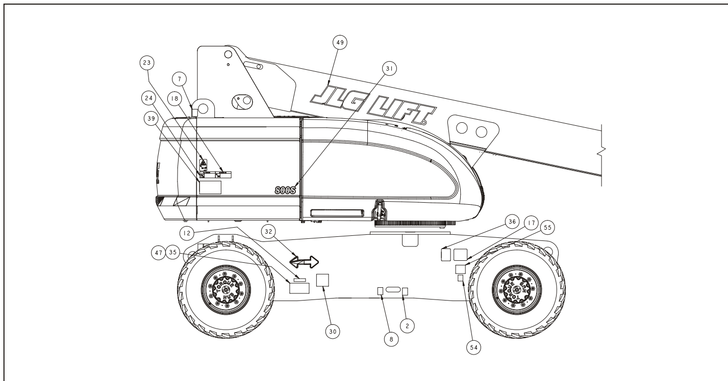
图4-7. 标志位置 - 第1页, 共5页
