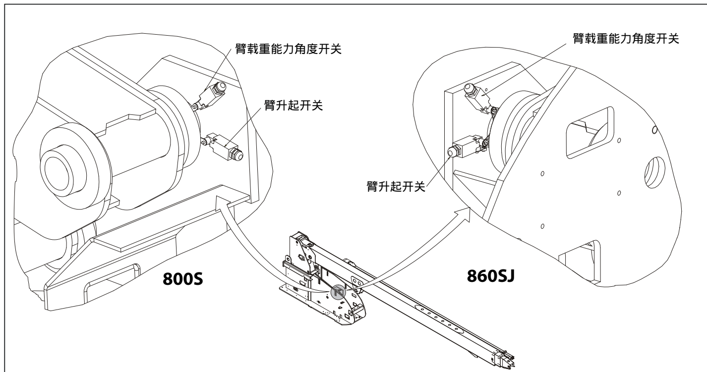
图 2-7. 限位和停止开关 - 第 1 页, 共 2 页
