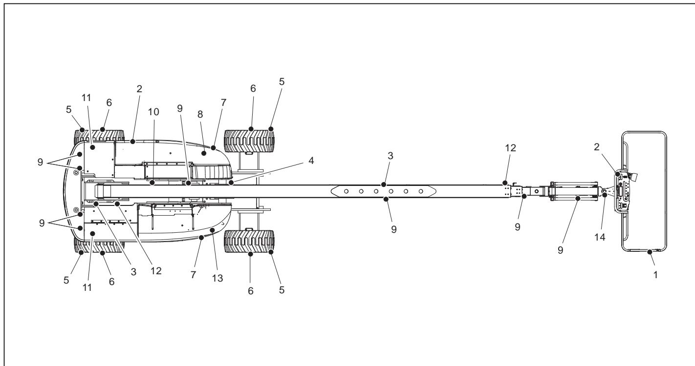
图 2-3. 日常巡视检查 - 第 1 页，共 2 页
