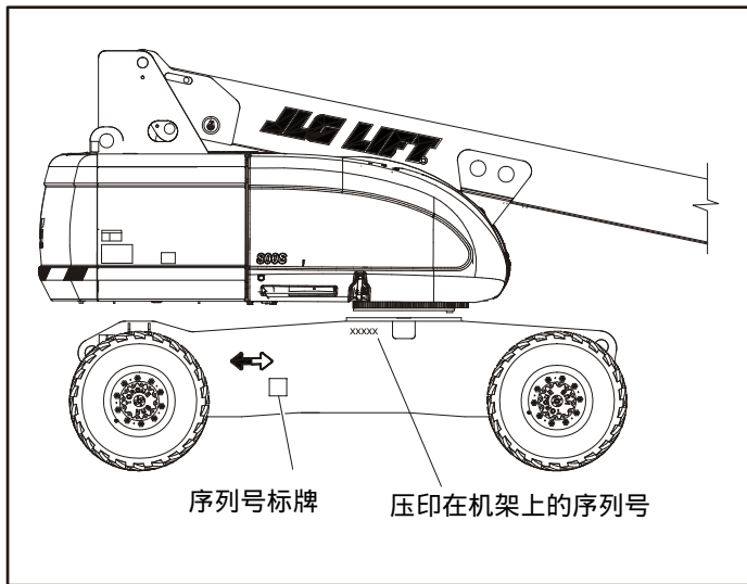
图 6-1. 序列号位置
